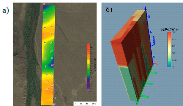
Рис. 2. а) Наложение на космоснимок карты кажущегося удельного сопротивления, построенной по результатам съемки ЭМЗВП; б) распределение удельного электрического сопротивления в объеме
