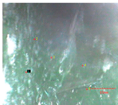
Рис. 2. Особенности распределения элементов (мас. %) в яблочно-зеленом флюорите
