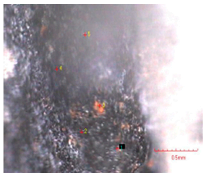
Рис. 3. Особенности распределения элементов (мас. %) в чернильно-фиолетовом флюорите
